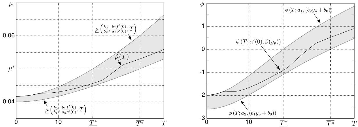
Figure 4 – Gauche . Illustration de la condition de stabilité correspondant aux stratégies de lutte biologique dans le plan (T, \mu) . La solution sans nuisible est asymptotiquement stable pour les couples (T, \mu) au dessus de la zone grisée et instable en dessous. L'analyse ne permet pas de conclure dans la zone grisée à cause des conditions de type secteur qui bornent certaines non-linéarités du modèle. Droite . Illustration du taux de convergence de la densité de nuisibles moyenné sur une période T , \phi , en fonction de la stratégie d'introduction déterminée par T pour un \mu fixé. Reproduit depuis (Nundloll et al., 2010a).
